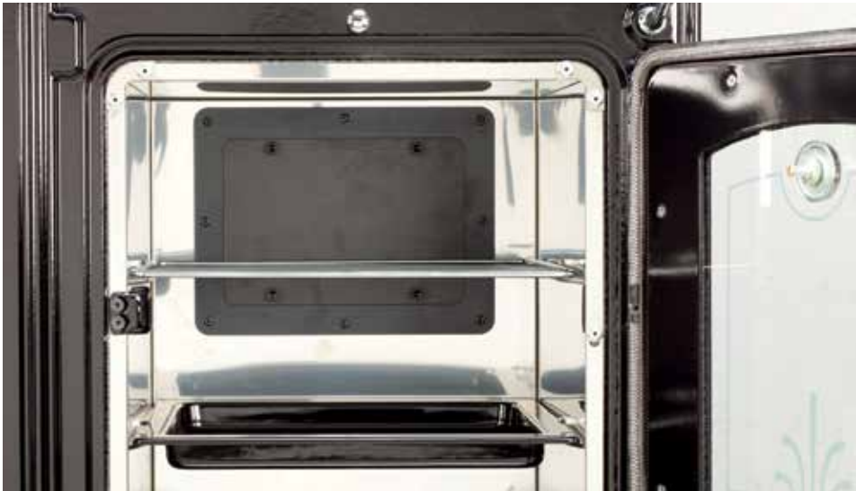
Todos los hornos inoxidables con escotilla de acceso a la salida de humos para facilitar la limpieza del conducto (sistema patentado por Lacunza)
